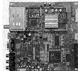
ケンテックのDTV/PVR一体型モジュール
